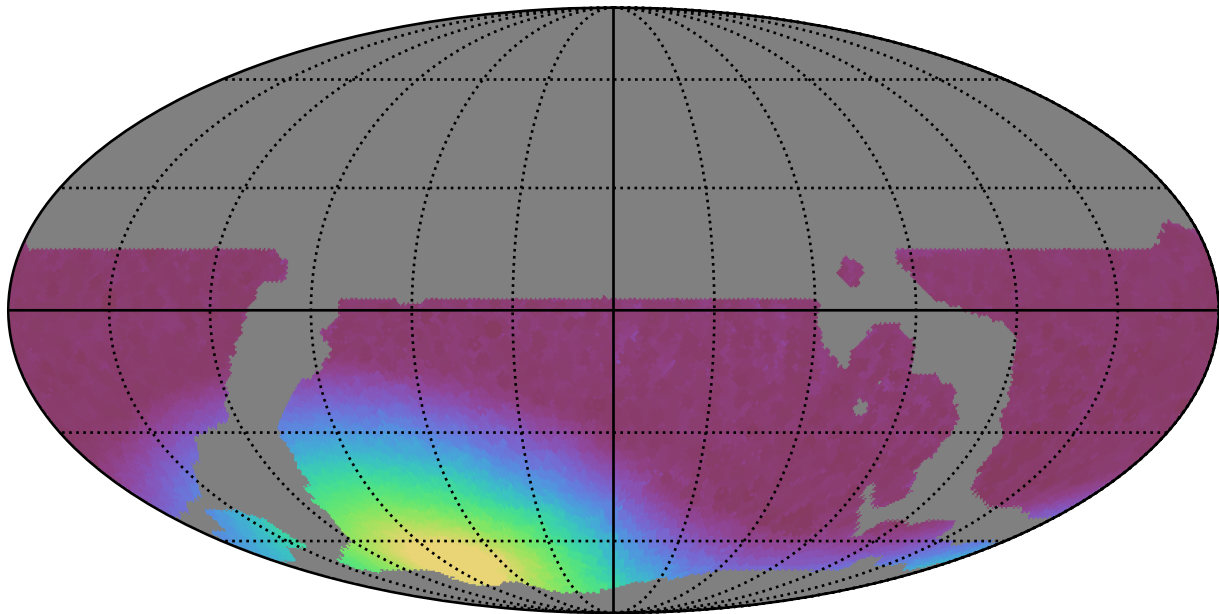
weather_cloudso6v3.4_10yrs WFD y band: Min moonDistance
