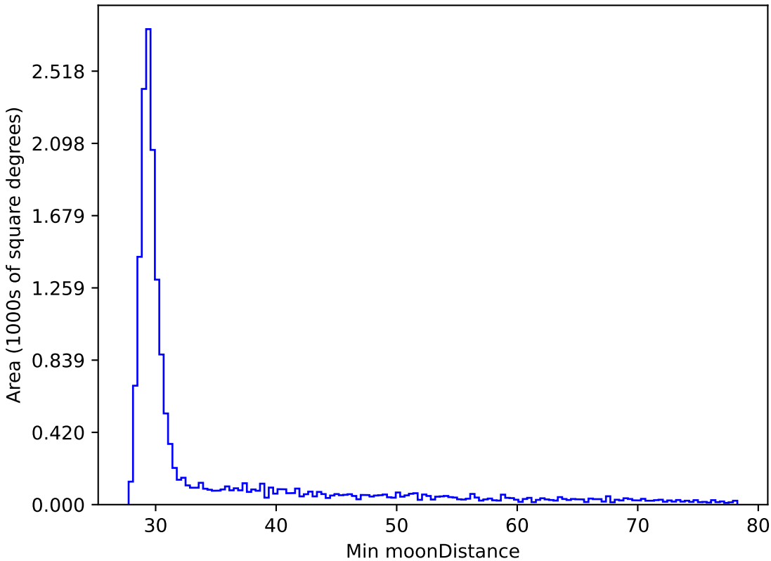
weather_cloudso6v3.4_10yrs WFD y band: Min moonDistance
