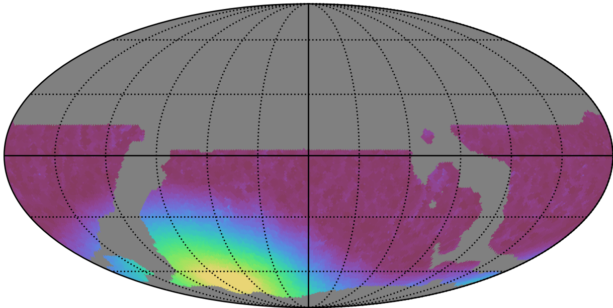
weather_cloudso6v3.4_10yrs WFD i band: Min moonDistance
