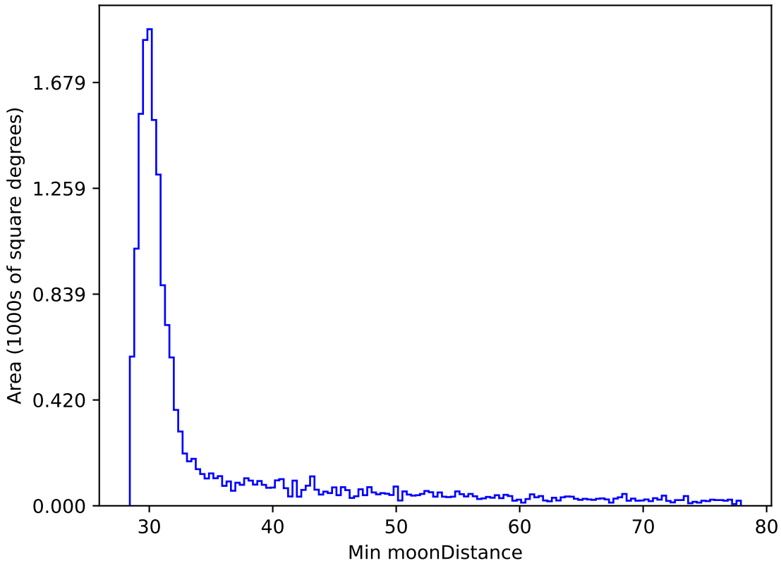
weather_cloudso6v3.4_10yrs WFD i band: Min moonDistance
