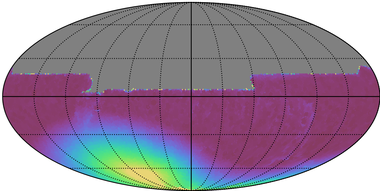
weather_cloudso6v3.4_10yrs All sky y band: Min moonDistance
