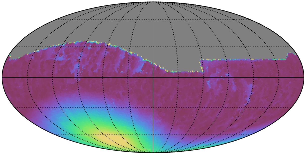
weather_cloudso6v3.4_10yrs All sky i band: Min moonDistance
