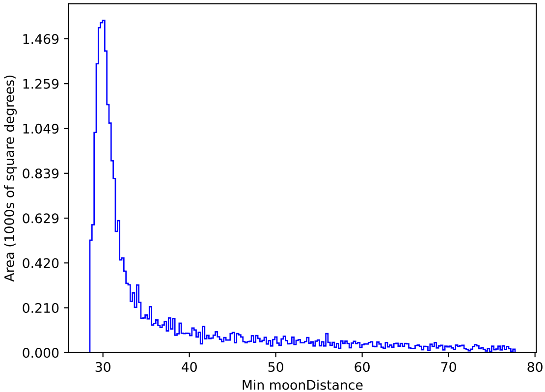
weather_cloudso6v3.4_10yrs All sky i band: Min moonDistance
