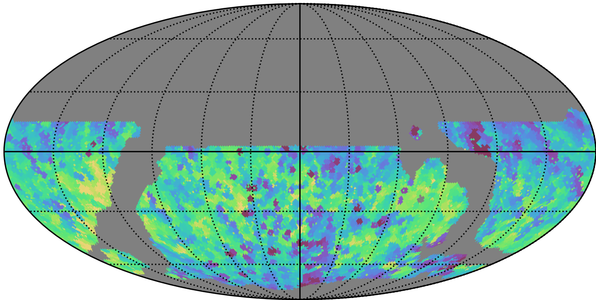
weather_cloudso6v3.4_10yrs WFD y band: Min fiveSigmaDepth
