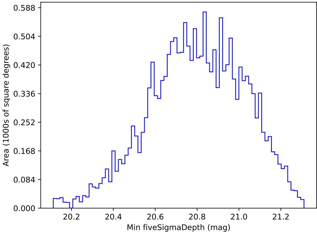
weather_cloudso6v3.4_10yrs WFD y band: Min fiveSigmaDepth
