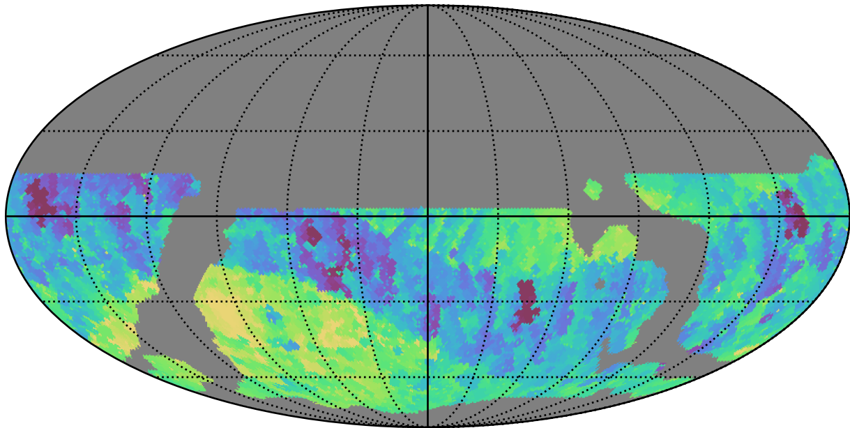
weather_cloudso6v3.4_10yrs WFD i band: Min fiveSigmaDepth
