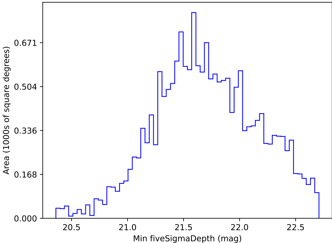
weather_cloudso6v3.4_10yrs WFD i band: Min fiveSigmaDepth
