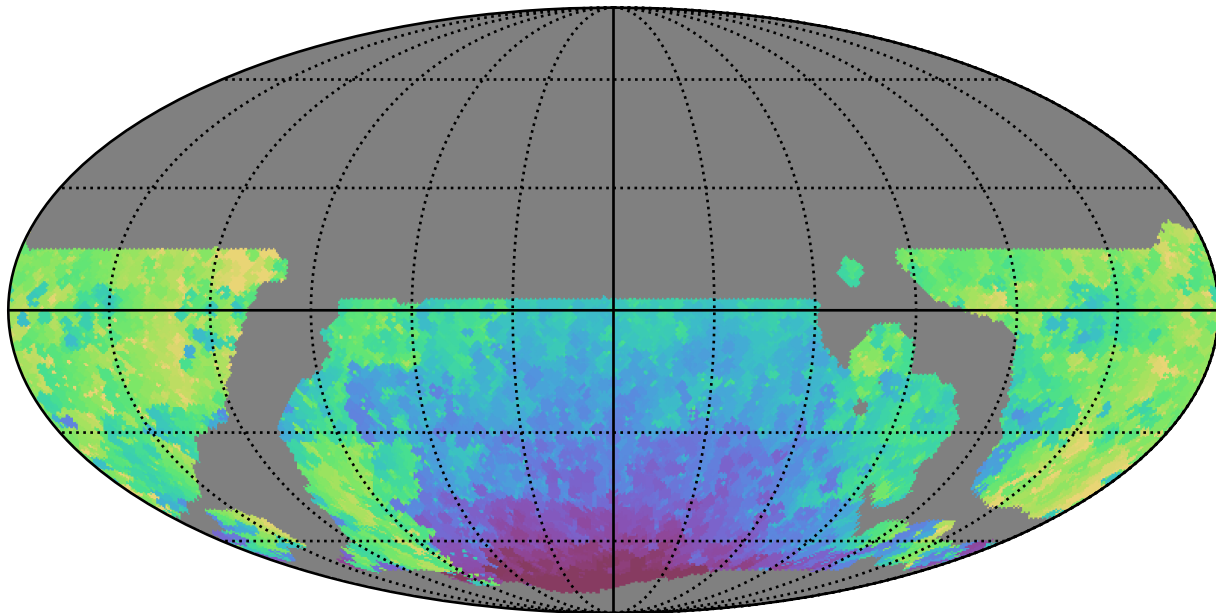
weather_cloudso6v3.4_10yrs WFD y band: Min HA
