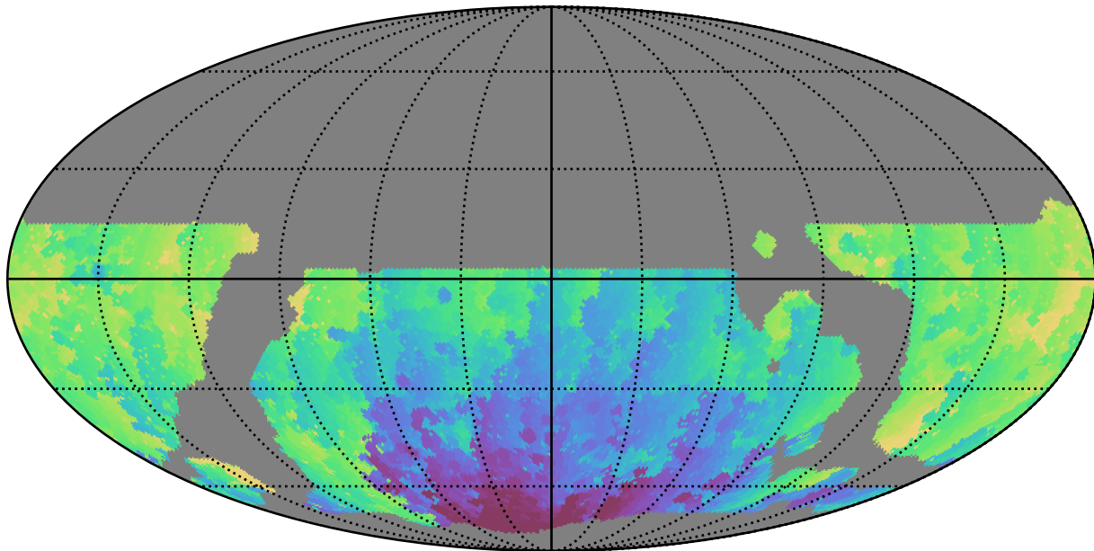
weather_cloudso6v3.4_10yrs WFD u band: Min HA
