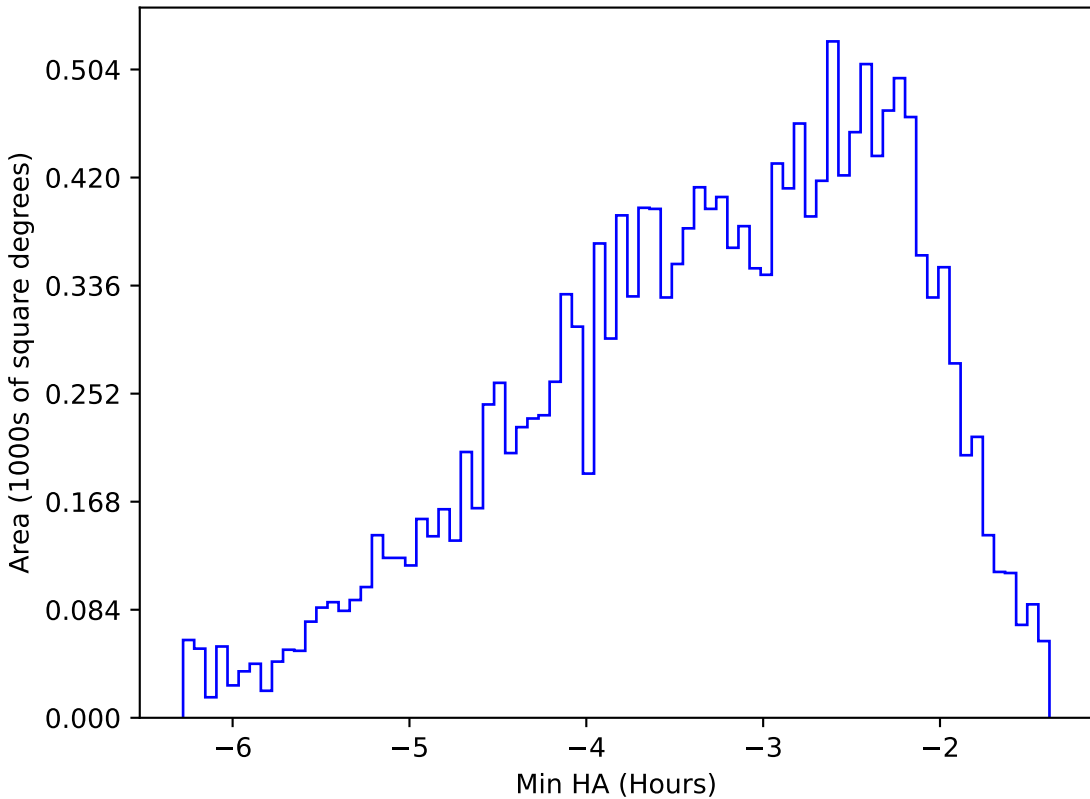
weather_cloudso6v3.4_10yrs WFD u band: Min HA
