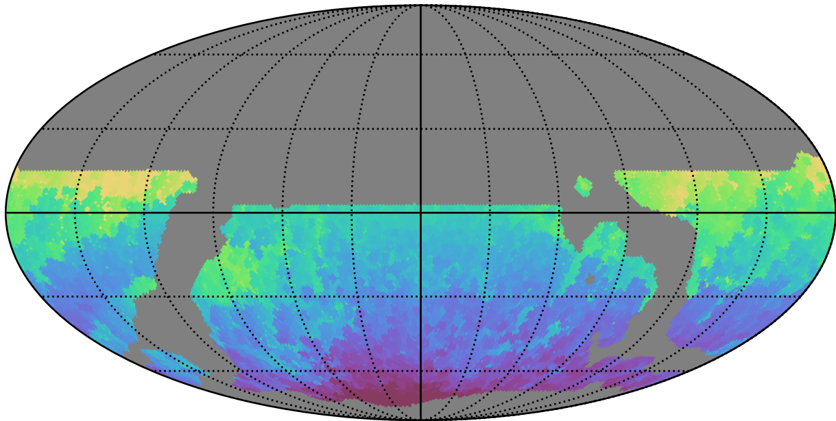
weather_cloudso6v3.4_10yrs WFD i band: Min HA
