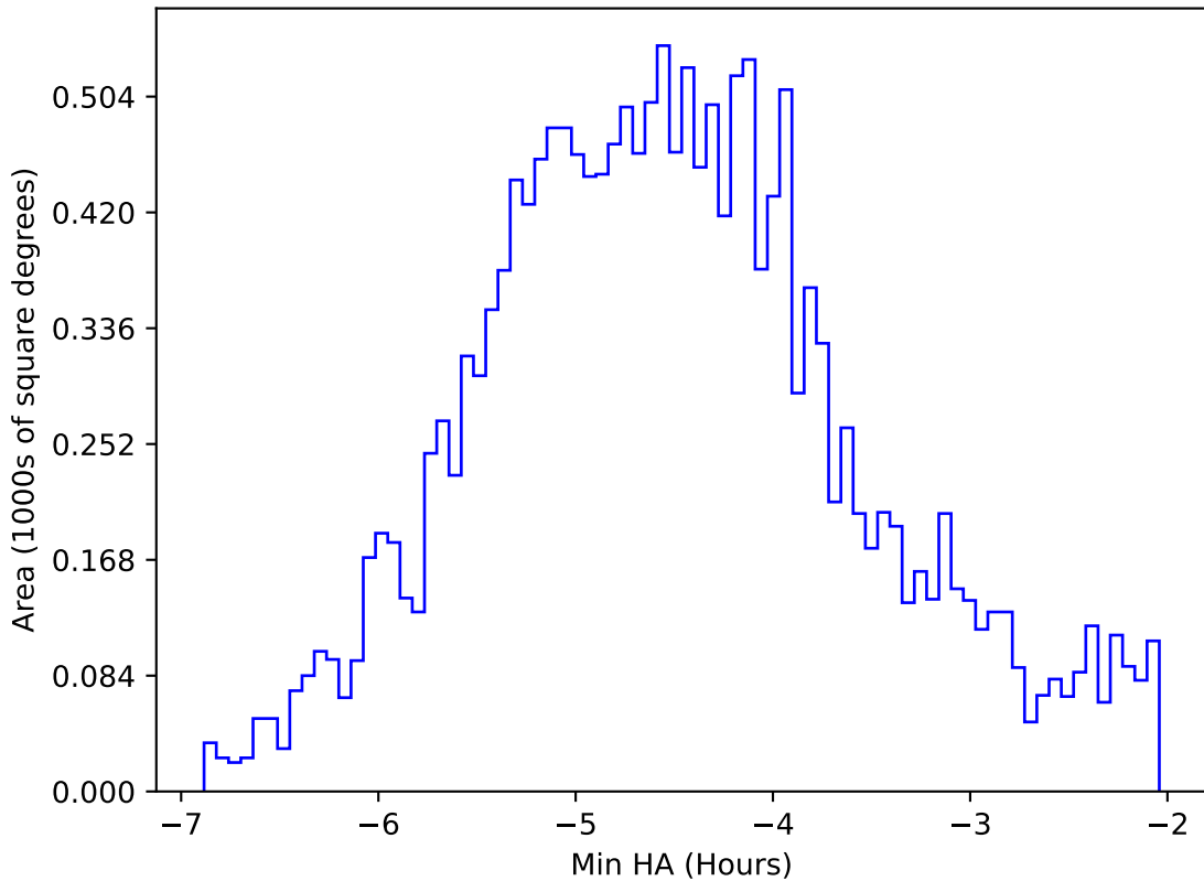
weather_cloudso6v3.4_10yrs WFD i band: Min HA
