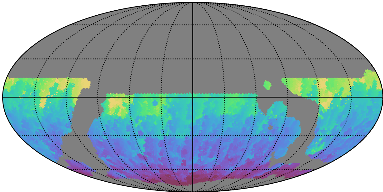
weather_cloudso6v3.4_10yrs WFD g band: Min HA
