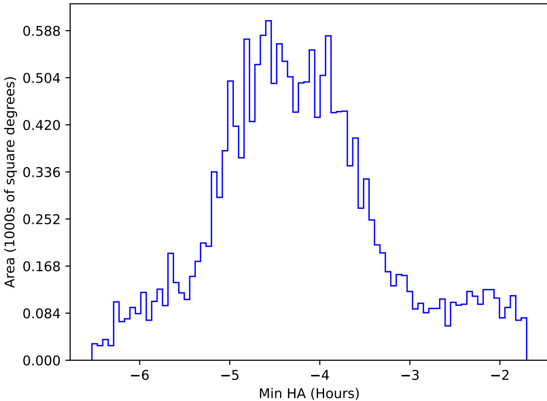
weather_cloudso6v3.4_10yrs WFD g band: Min HA
