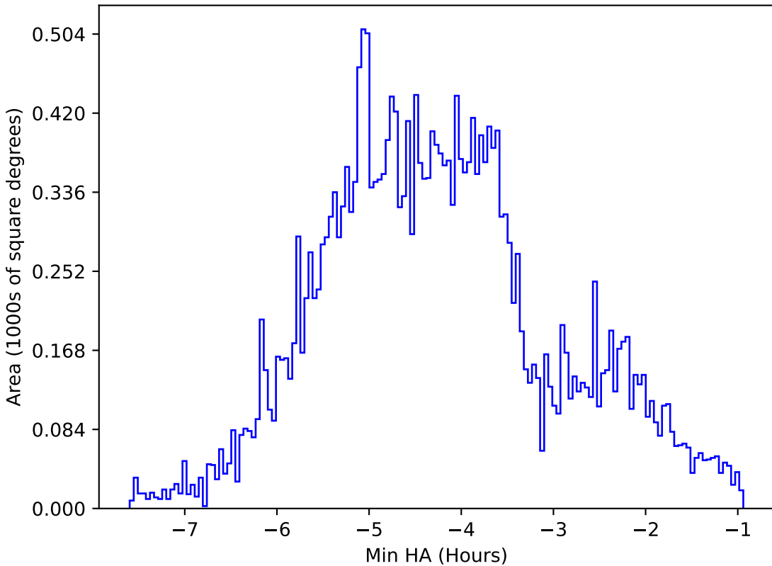
weather_cloudso6v3.4_10yrs All sky z band: Min HA
