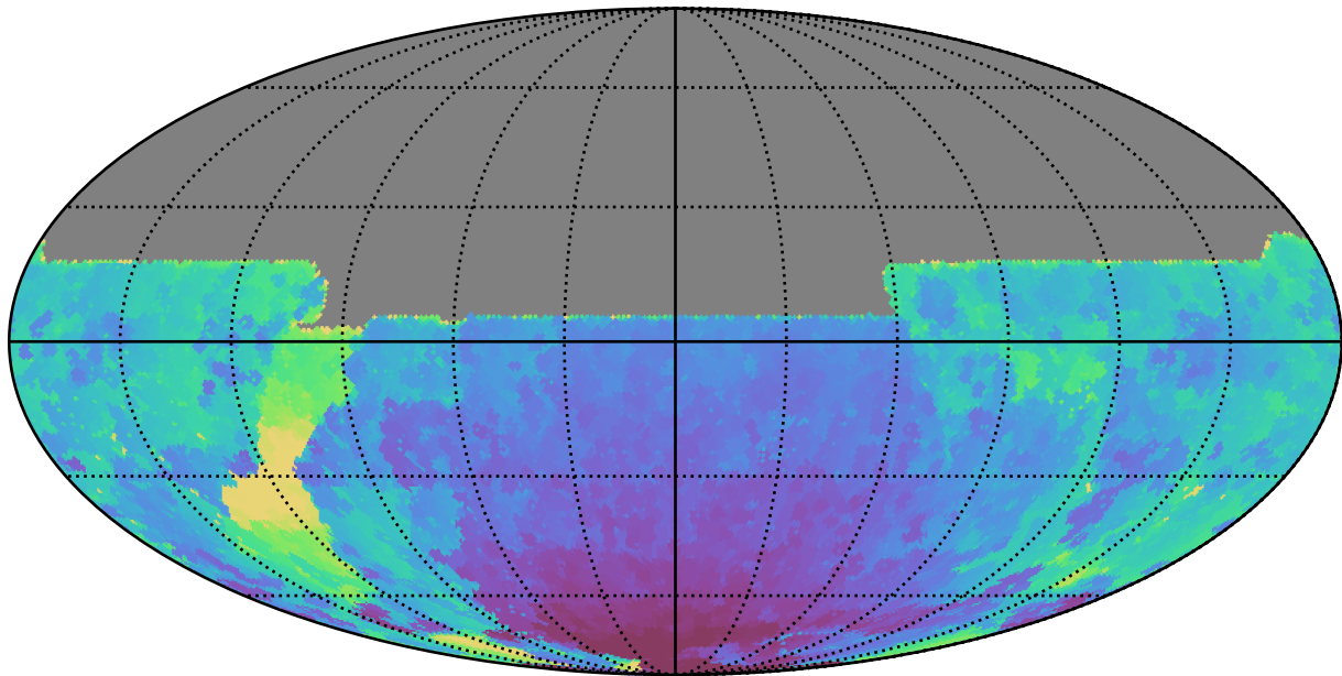
weather_cloudso6v3.4_10yrs All sky y band: Min HA
