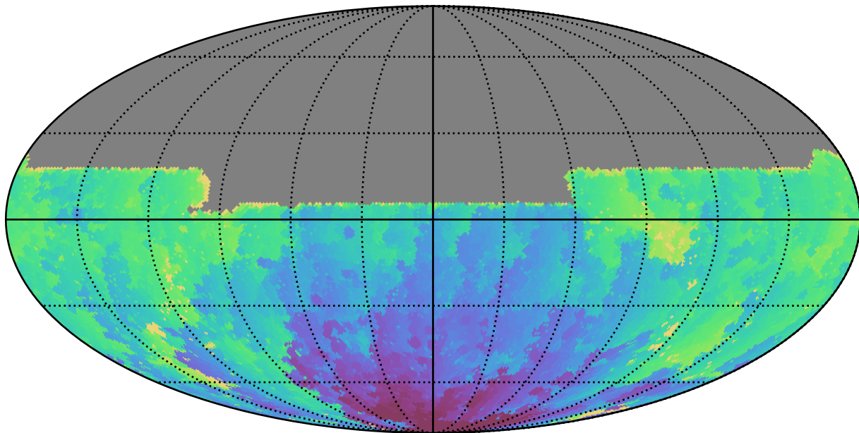
weather_cloudso6v3.4_10yrs All sky u band: Min HA
