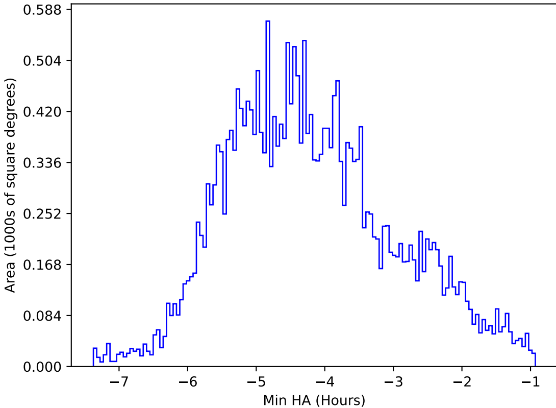
weather_cloudso6v3.4_10yrs All sky r band: Min HA
