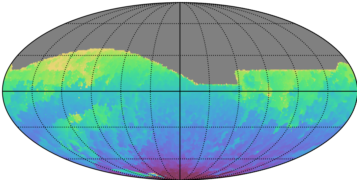
weather_cloudso6v3.4_10yrs All sky i band: Min HA
