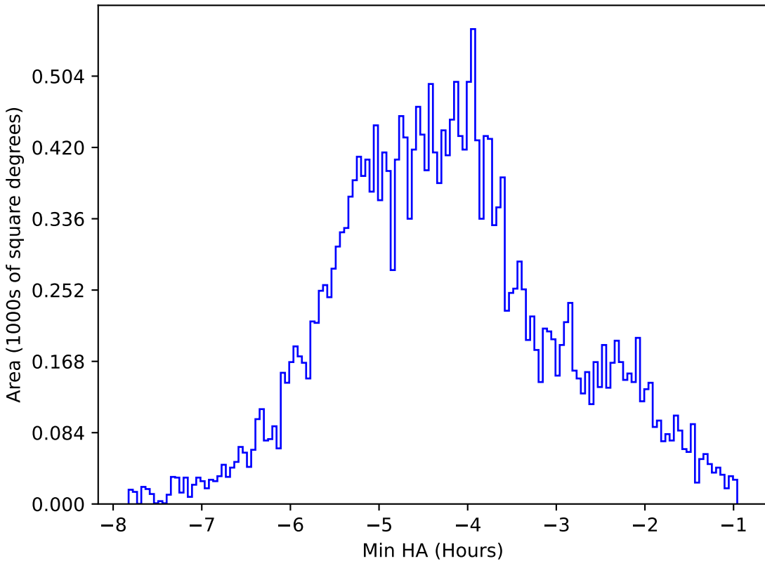
weather_cloudso6v3.4_10yrs All sky i band: Min HA
