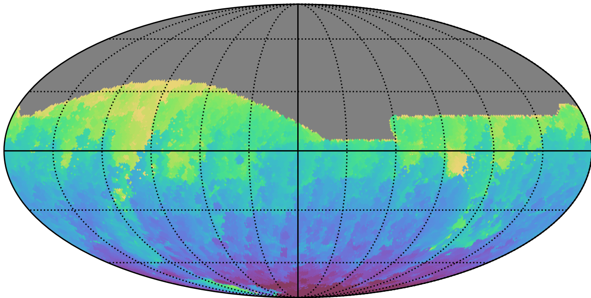
weather_cloudso6v3.4_10yrs All sky g band: Min HA
