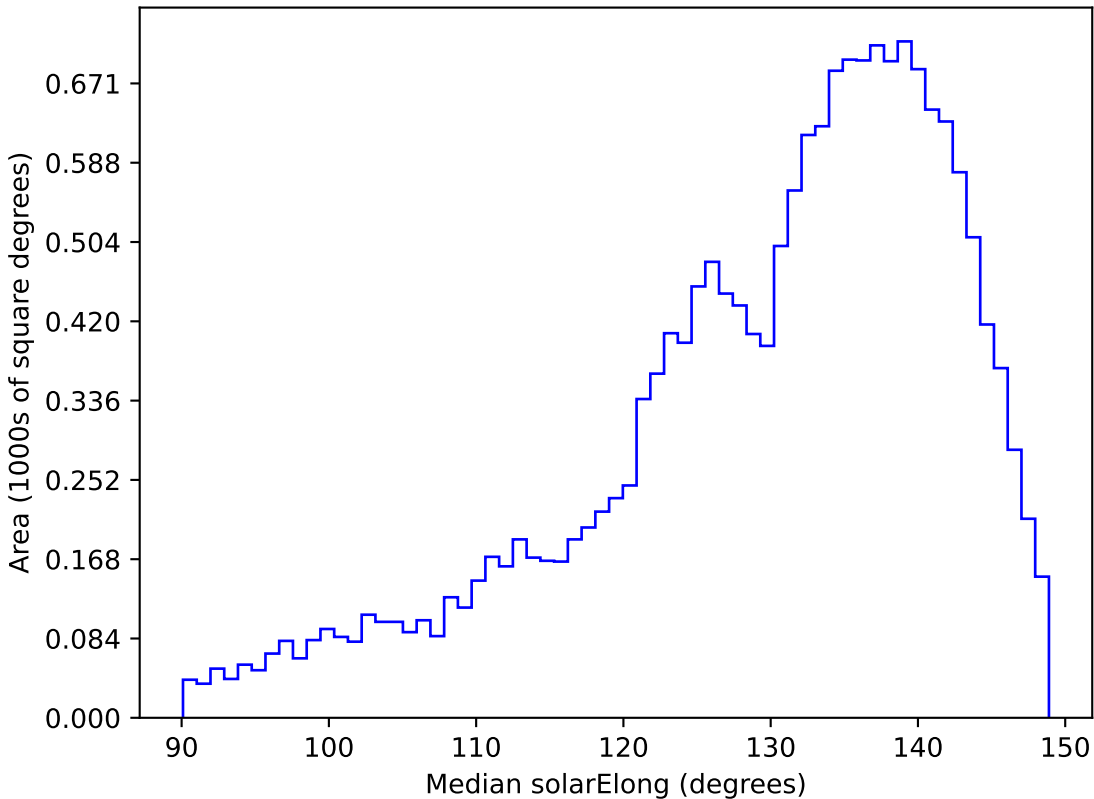
weather_cloudso6v3.4_10yrs WFD y band: Median solarElong
