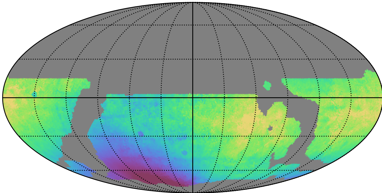
weather_cloudso6v3.4_10yrs WFD i band: Median solarElong
