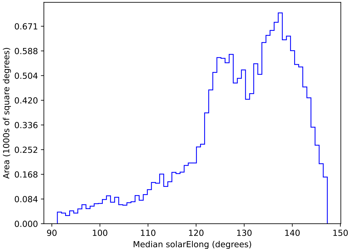
weather_cloudso6v3.4_10yrs WFD i band: Median solarElong
