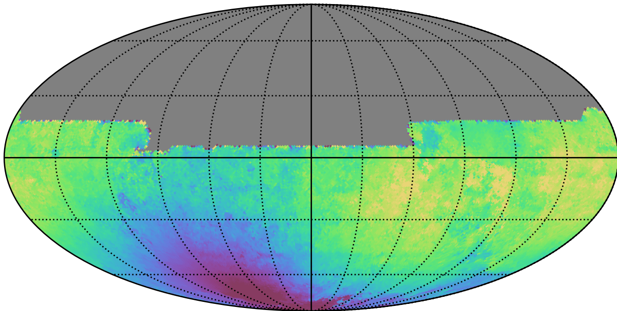
weather_cloudso6v3.4_10yrs All sky y band: Median solarElong
