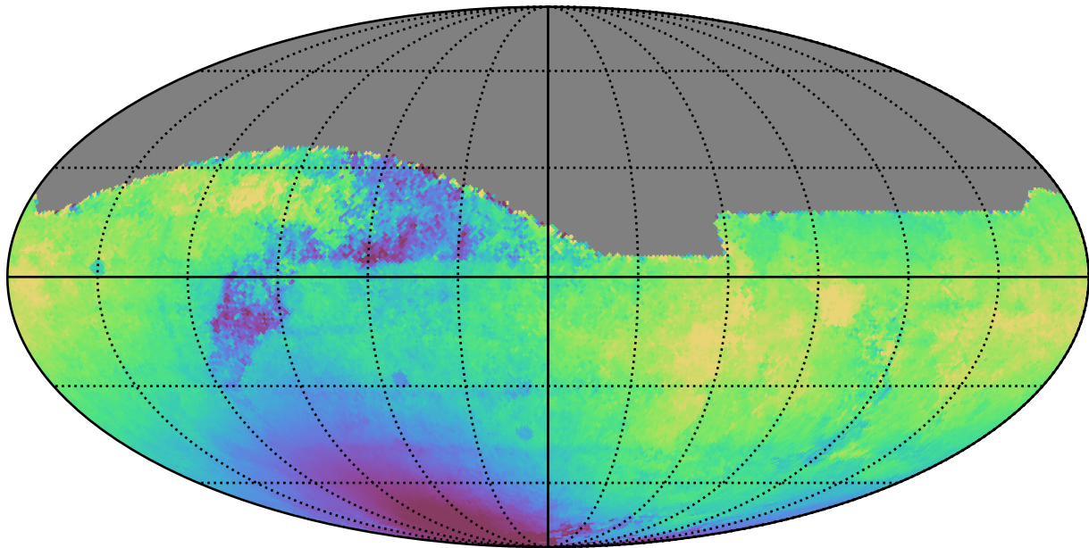
weather_cloudso6v3.4_10yrs All sky i band: Median solarElong
