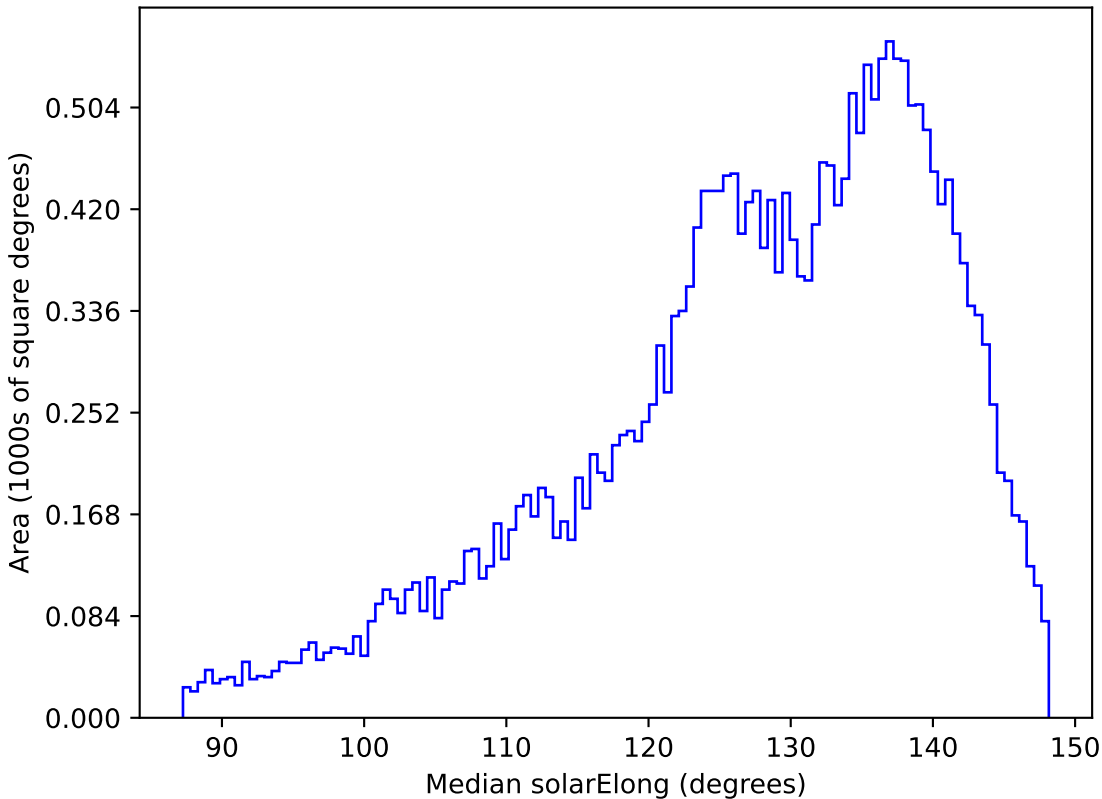
weather_cloudso6v3.4_10yrs All sky i band: Median solarElong
