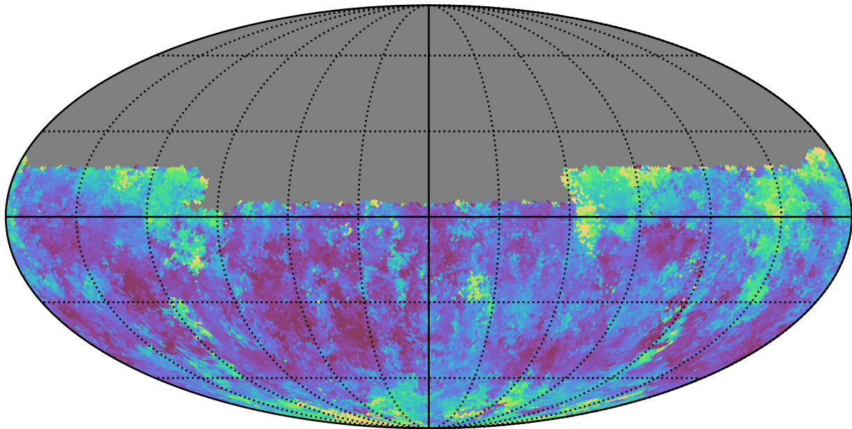
weather_cloudso6v3.4_10yrs Yr 1 y band: Median seeingGeom
