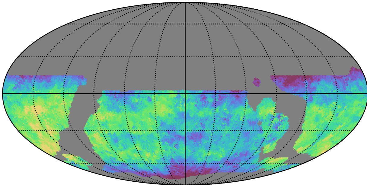
weather_cloudso6v3.4_10yrs WFD u band: Median saturation_mag
