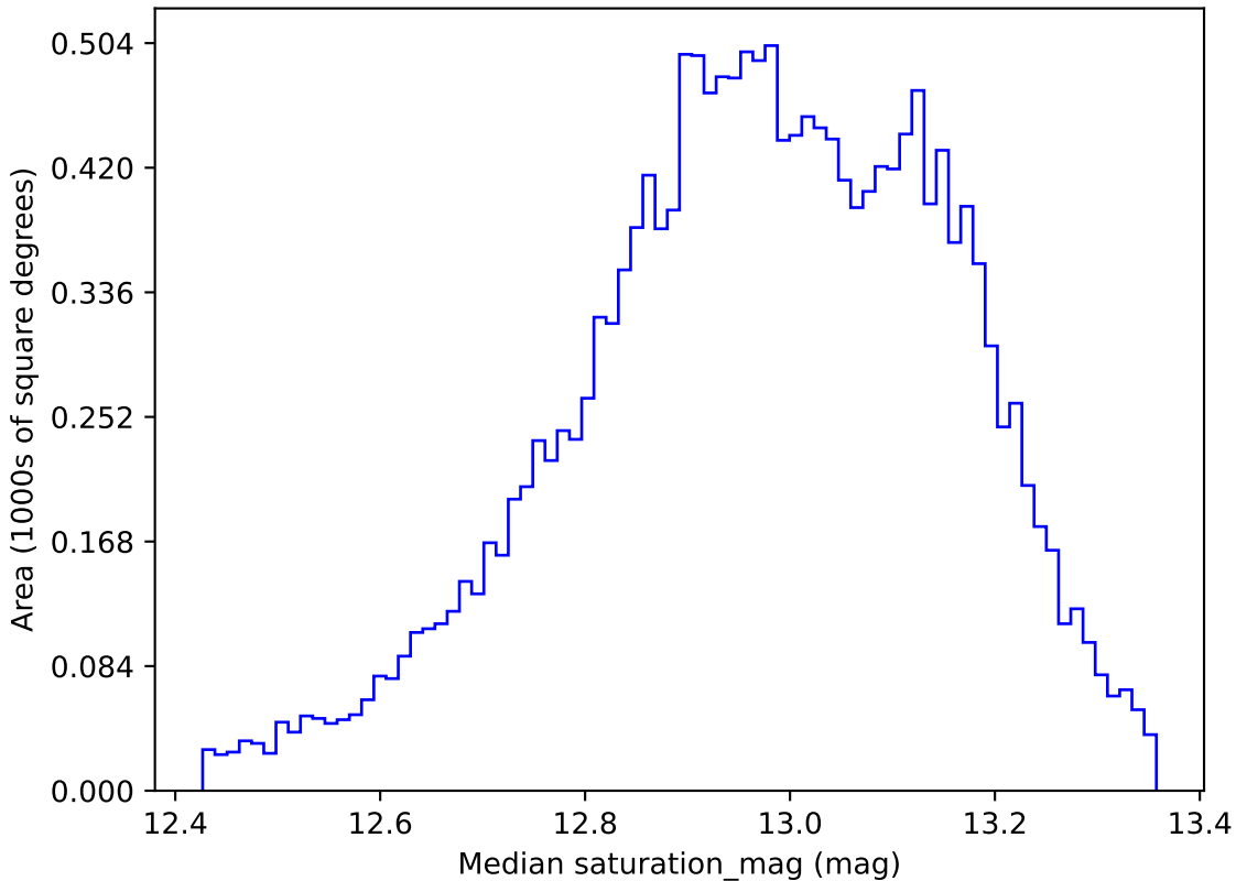
weather_cloudso6v3.4_10yrs WFD u band: Median saturation_mag
