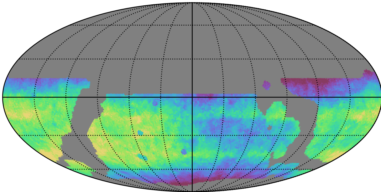
weather_cloudso6v3.4_10yrs WFD r band: Median saturation_mag
