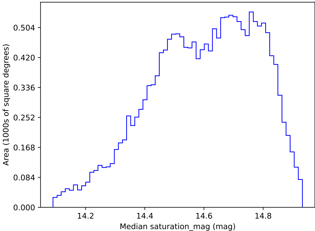
weather_cloudso6v3.4_10yrs WFD r band: Median saturation_mag
