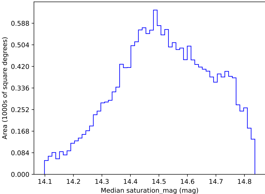
weather_cloudso6v3.4_10yrs WFD i band: Median saturation_mag
