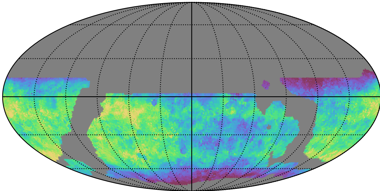
weather_cloudso6v3.4_10yrs WFD g band: Median saturation_mag
