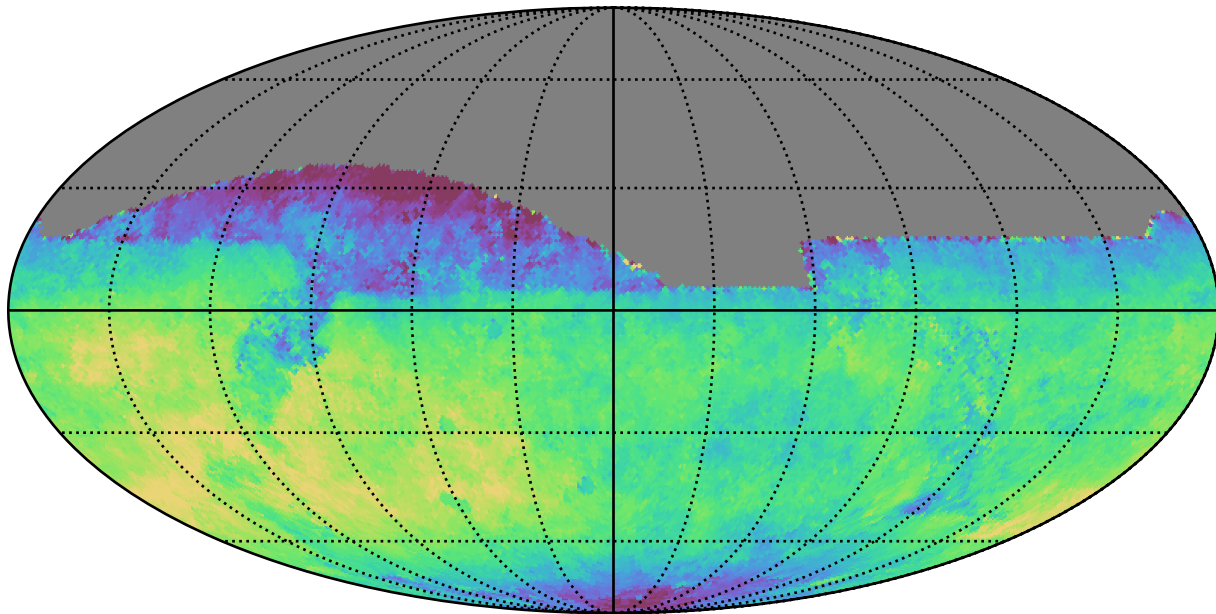
weather_cloudso6v3.4_10yrs All sky z band: Median saturation_mag
