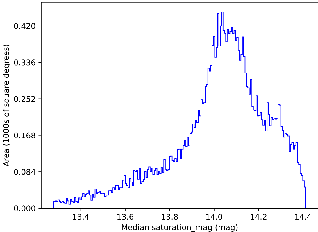
weather_cloudso6v3.4_10yrs All sky z band: Median saturation_mag
