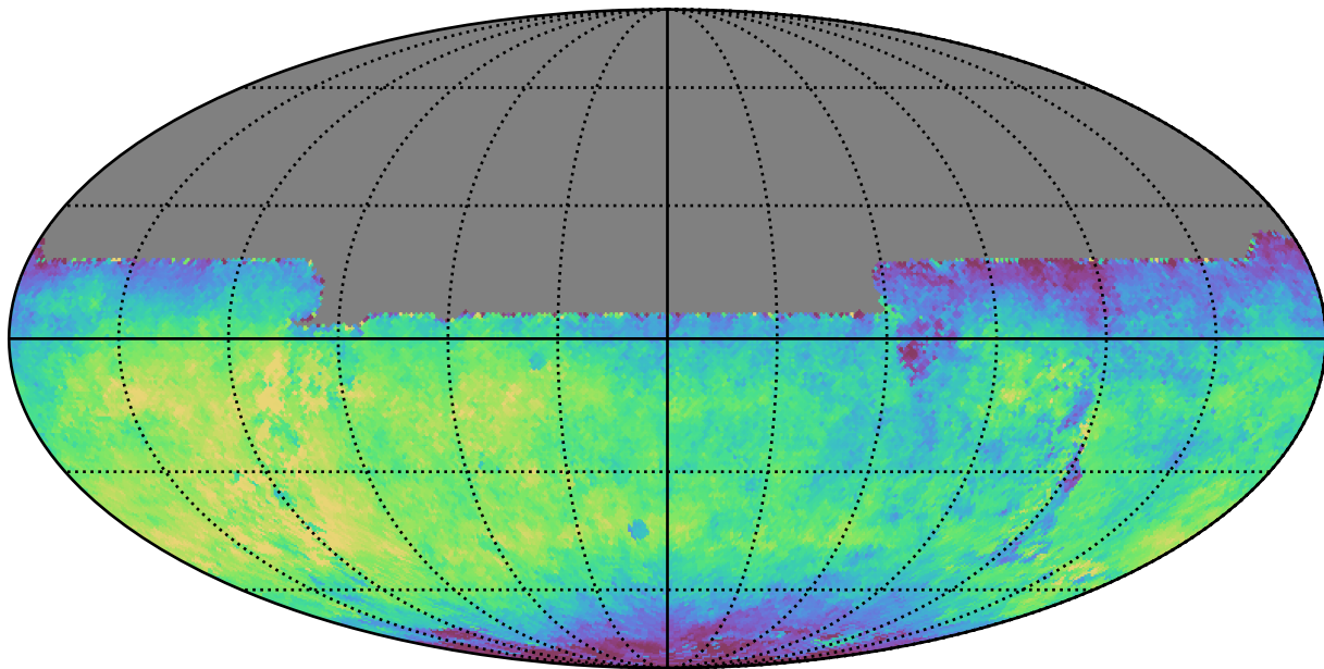
weather_cloudso6v3.4_10yrs All sky y band: Median saturation_mag
