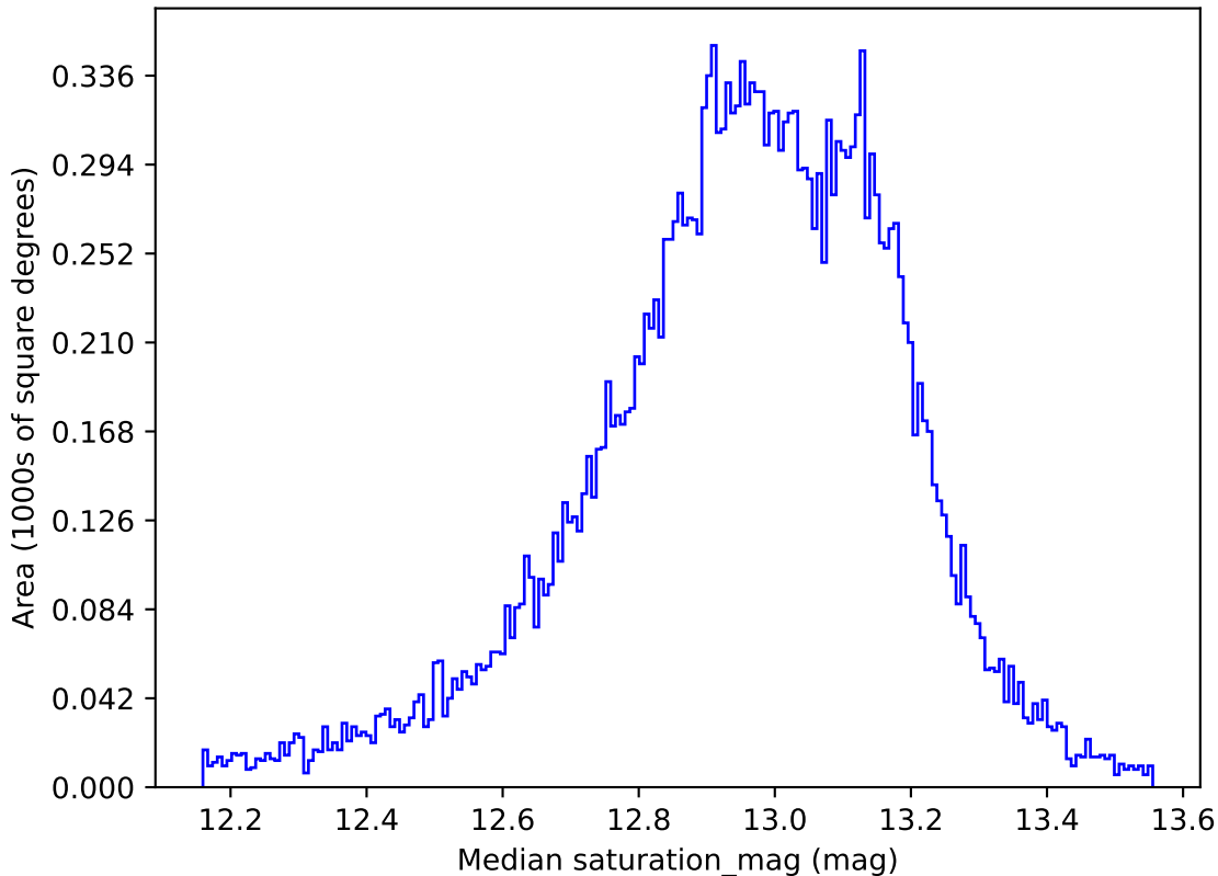
weather_cloudso6v3.4_10yrs All sky u band: Median saturation_mag
