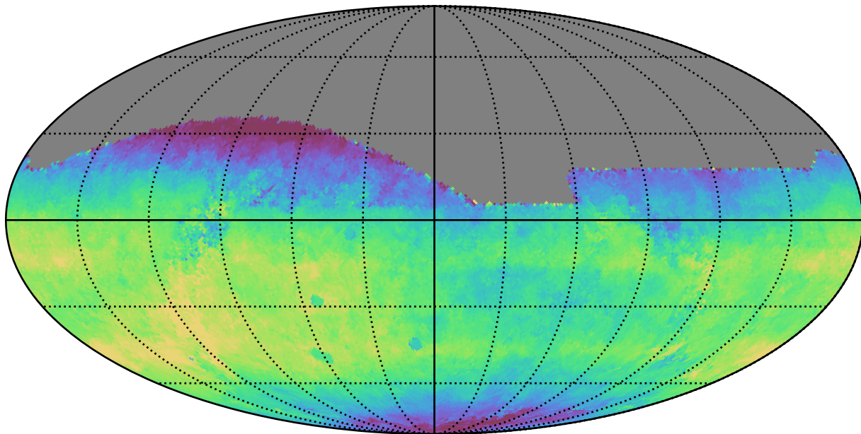
weather_cloudso6v3.4_10yrs All sky r band: Median saturation_mag
