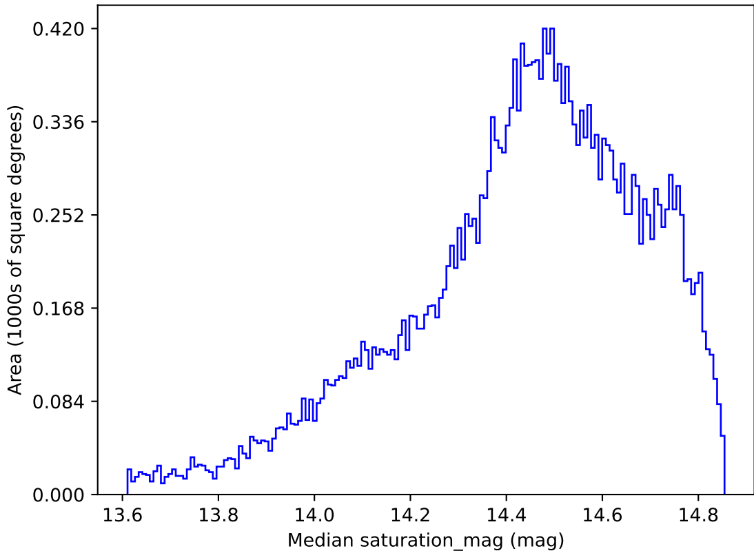
weather_cloudso6v3.4_10yrs All sky i band: Median saturation_mag
