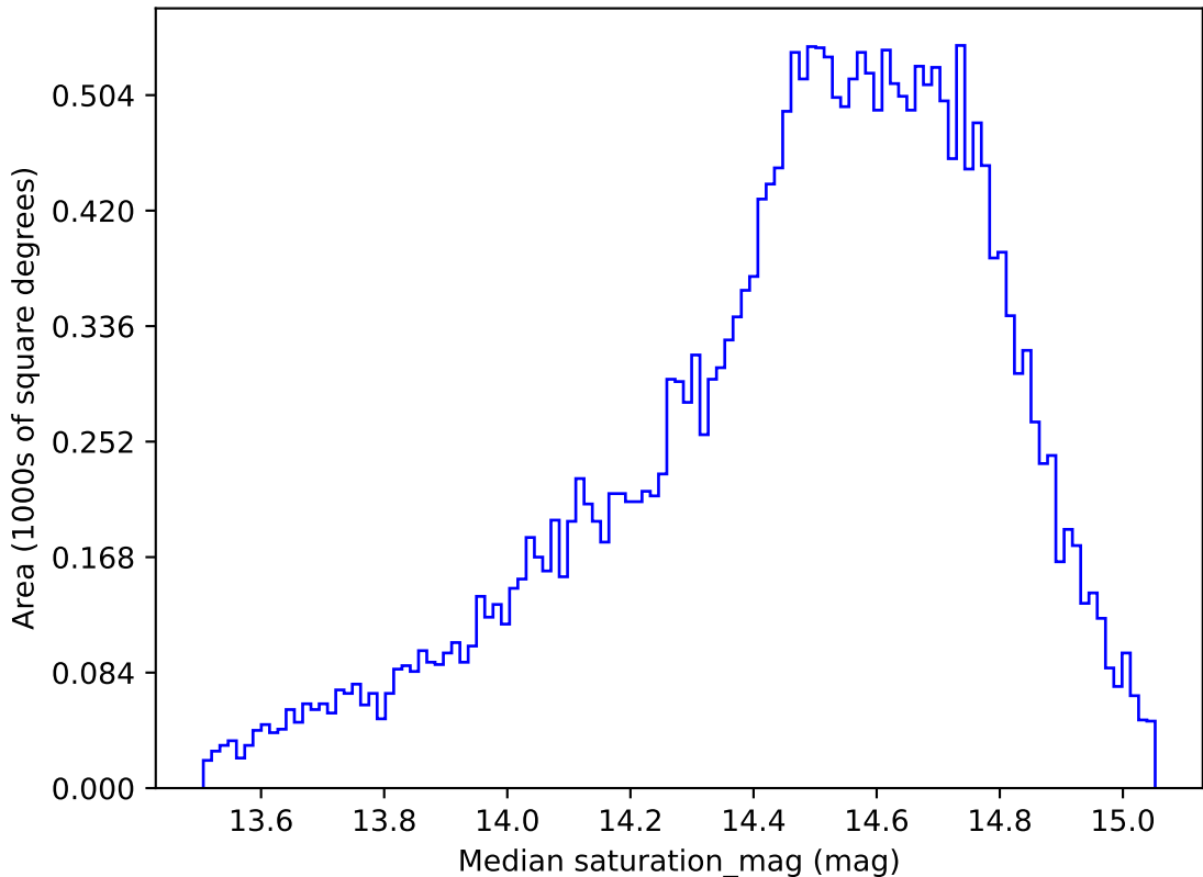
weather_cloudso6v3.4_10yrs All sky g band: Median saturation_mag
