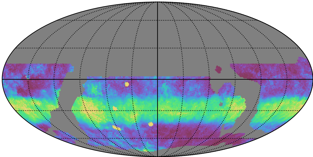
weather_cloudso6v3.4_10yrs WFD y band: Median normairmass
