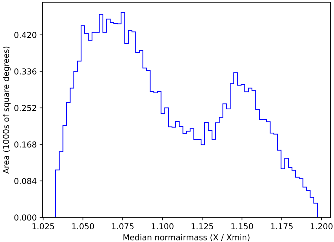
weather_cloudso6v3.4_10yrs WFD y band: Median normairmass
