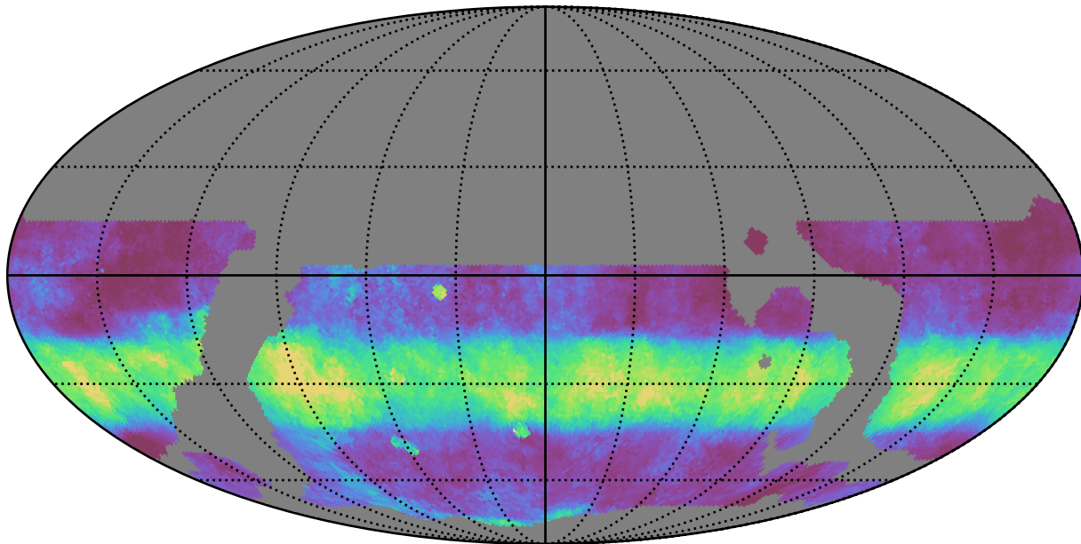
weather_cloudso6v3.4_10yrs WFD i band: Median normairmass
