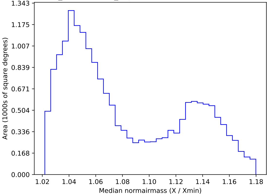
weather_cloudso6v3.4_10yrs WFD i band: Median normairmass
