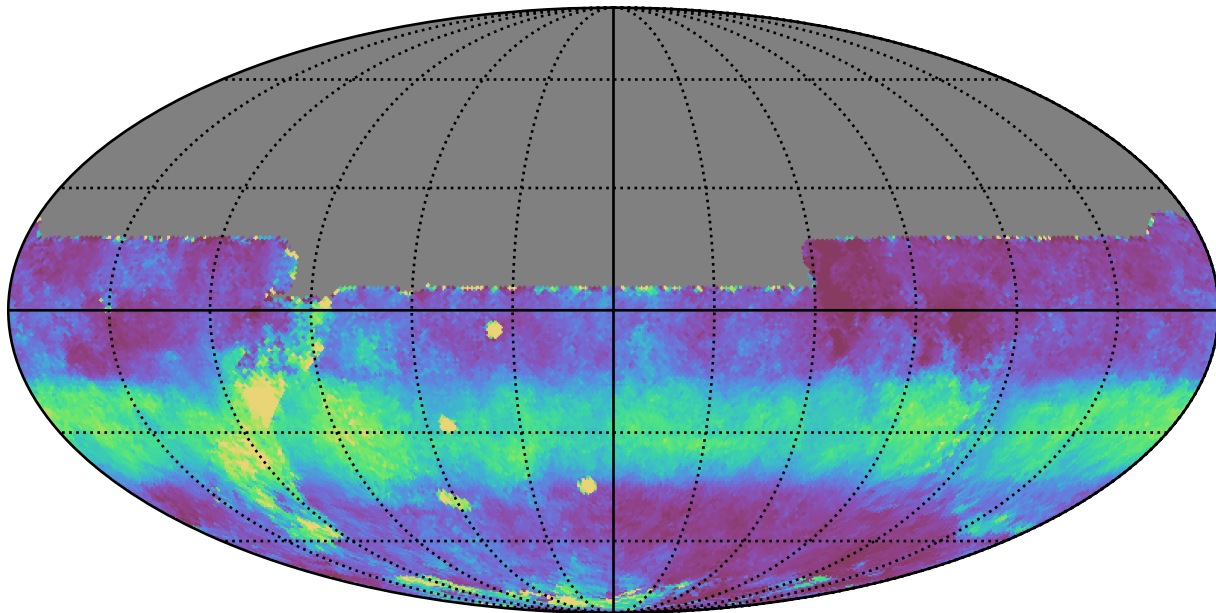
weather_cloudso6v3.4_10yrs All sky y band: Median normairmass
